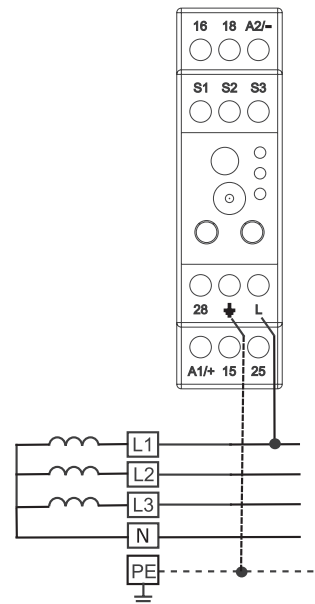
C) 3P 4W AC SYSTEM
